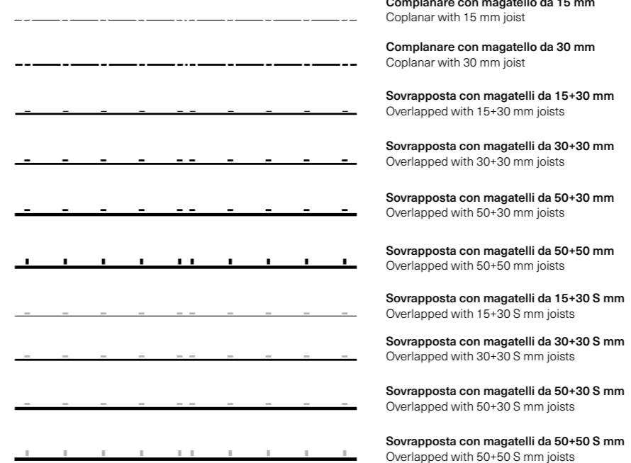
CONFIGURAZIONE STRUTTURA METALLICA METAL STRUCTURE CONFIGURATION
