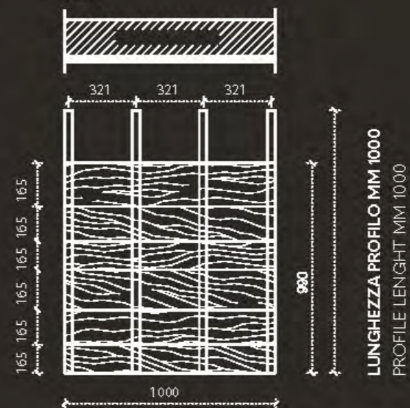
SCHEMA DI MONTAGGIO VERTICALE VERTICAL ASSEMBLY DIAGRAM EXAMPLE
